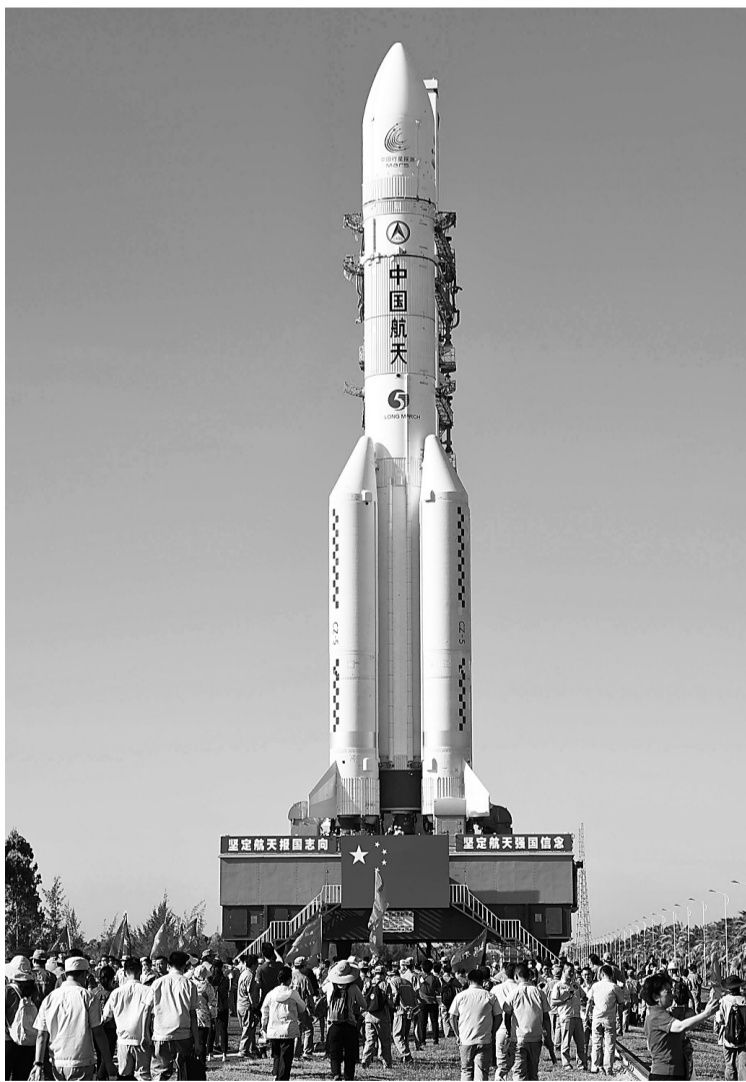
长征五号遥四运载火箭垂直转运至发射区
